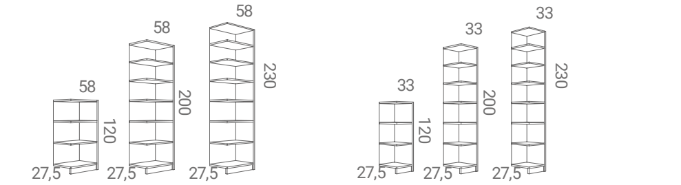
TILLBYGGNADSEKTION LT12058/LT20058/LT23058 TILLBYGGNADSEKTION LT12033/LT20033/LT23033
