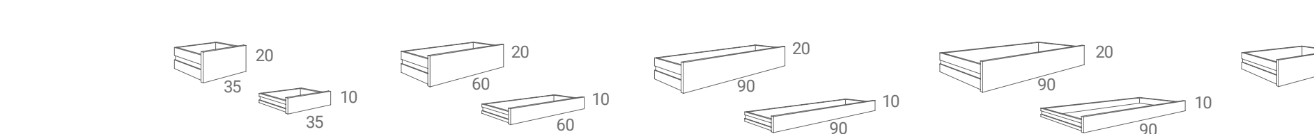
LÅDA LL2035/ LL1035 LÅDA LL2060/ LL1060 LÅDA LL2090/ LL1090 LÅDA TILL UNDERDEL LL2090u/ LL1090u LÅDA TILL UNDERDEL LL2060u/ LL1060u
