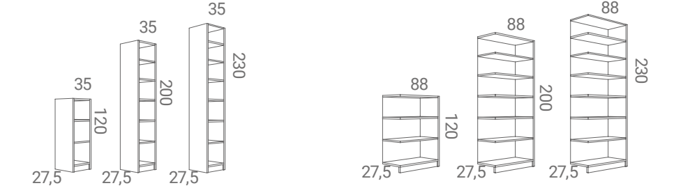
GRUNDSEKTION LG12035/LG20035/LG23035 TILLBYGGNADSEKTION LT12088/LT20088/LT23088
