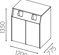
W3521 Hela dörrar för rullkärl 190 liter *
