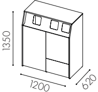
W3515 Hel dörr till vänster för rullkärl 140 l*, dörr ovan till för 2x60 l kärl och låd utdrag undertill till höger * *
