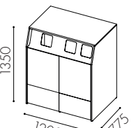
W3524 Dörr ovan till för 90 l kärl i enkelt inkast, 2x60 l i dubbelt inkast och låd utdrag undertill * *
