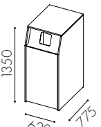
W3518 Hel dörr för rullkärl 190 liter *
