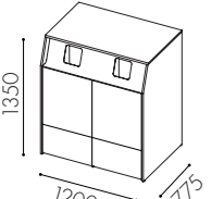
W3522 Dörr ovan till för 90 l kärl och låd utdrag undertill * *
