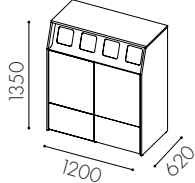
W3517 Dörr ovan till för 2x60 l kärl och låd utdrag undertill * *
