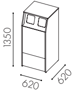
W3512 Dörr ovan till för 2x60 kärl och låd utdrag undertill * *
