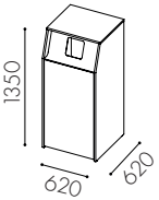
W3510 Hel dörr för rullkärl 140 liter *
