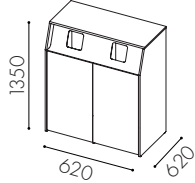
W3513 Hela dörrar för rullkärl 140 liter *
