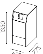
W3519 Dörr ovan till för 90 l kärl och låd utdrag undertill * *
