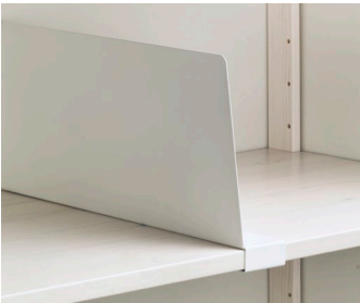
Hyllavskiljare H: 180 D: 250, 300, 400
