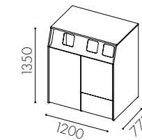
W3523 Hel dörr till vänster för rullkärl 190 l*, dörr ovan till för 2x60 l kärl och lådutdrag undertill till höger **
