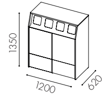
W3517 Dörr ovan till för 2x60 l kärl och lådutdrag undertill **
