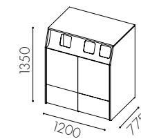
W3524 Dörr ovan till för 90 l kärl i enkelt inkast, 2x60 l i dubbelt inkast och lådutdrag undertill **
