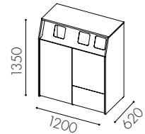
W3515 Hel dörr till vänster för rullkärl 140 l*, dörr ovan till för 2x60 l kärl och lådutdrag undertill till höger **
