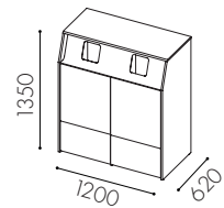
W3514 Dörr ovan till för 90 l kärl och lådutdrag undertill **
