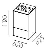
W3113 Dörr ovanpå för 2st 60l kärl och lådutdrag undertill *
